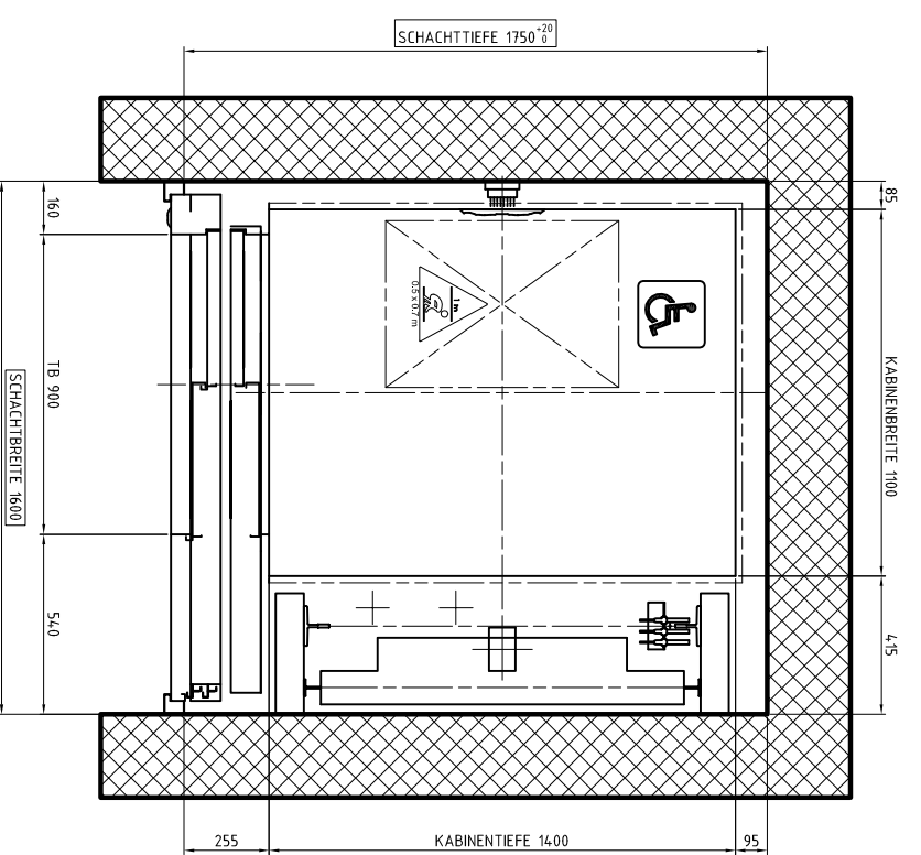
ZUGÄNGE SCHACHTGRUNDRISS
