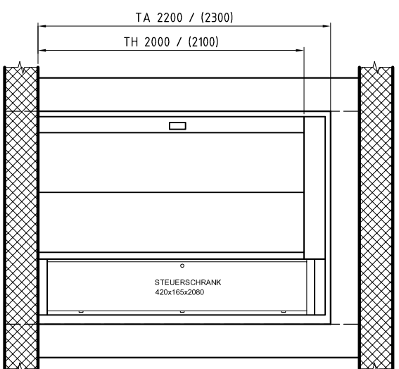
TÜRANSICHT STEUERSCHRANK
