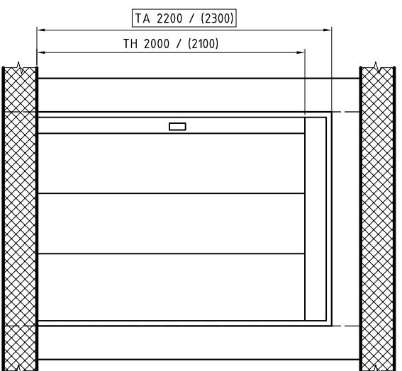
TÜRANSICHT
