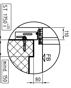
DETAIL Y
