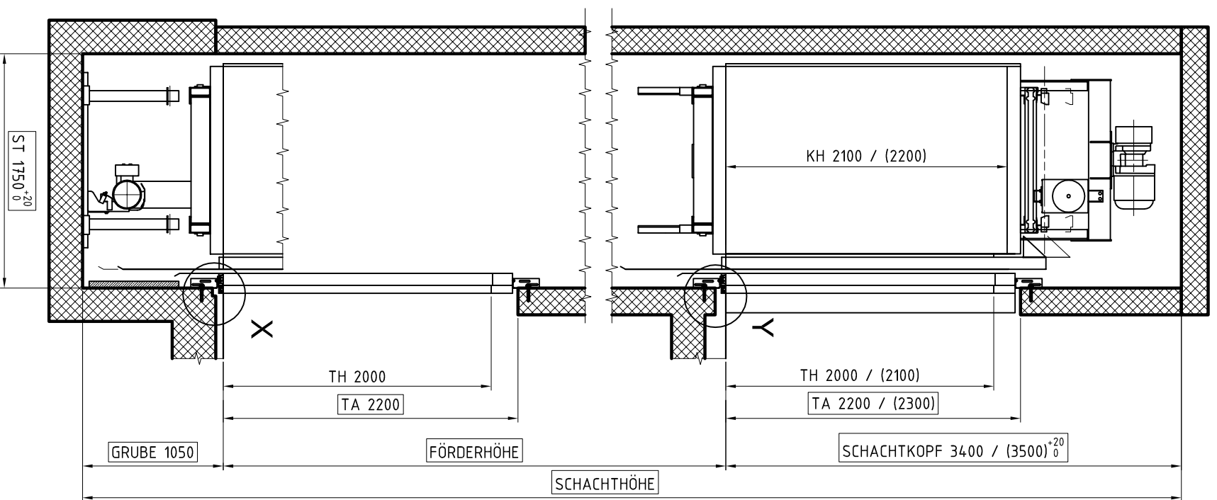
VERTIKALSCHNITT
